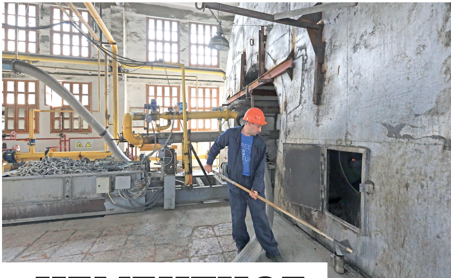
Рабочий берёт из печи пробу продукта высокотемпературного обжига.
