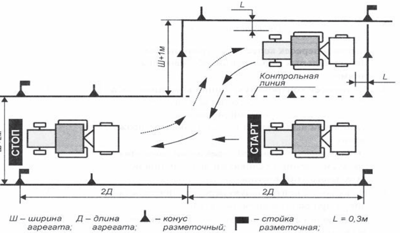
Рис. 16. Парковка СМ с прицепом задним ходом и выезд с парковочного места, параллельная парковка
