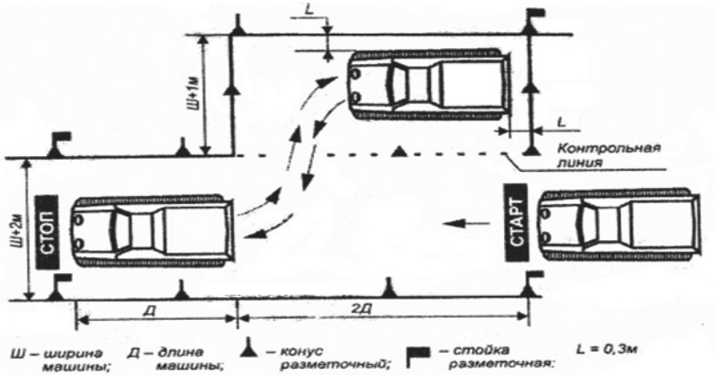
Рис. 15. Парковка СМ задним ходом и выезд с парковочного места, параллельная парковка
