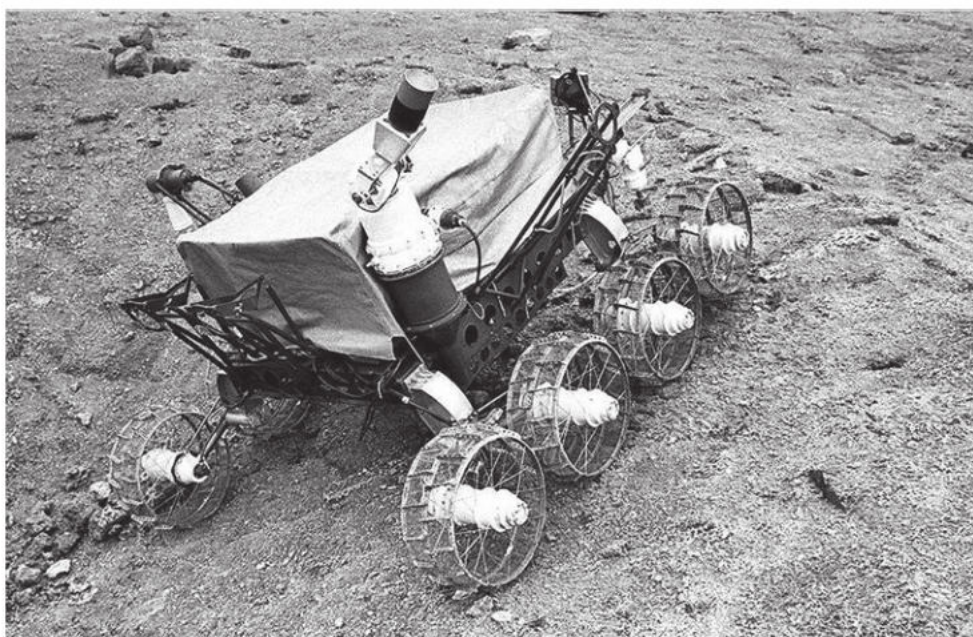
Испытание шасси лунохода на лунодроме под Симферополем.
